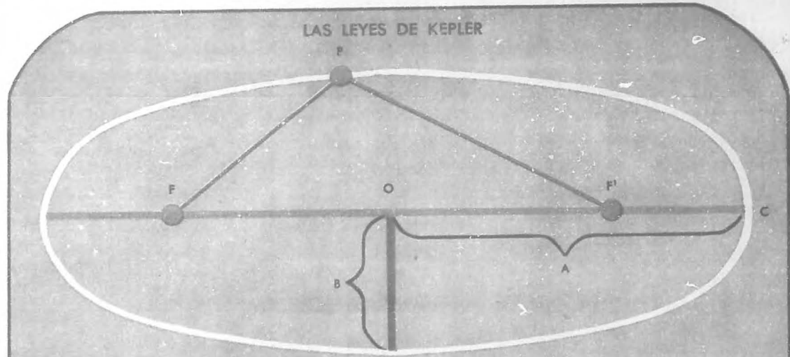
Geometría de la elipse Fig. 1
