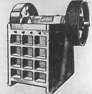
Trituradoras y Pulverizadoras LIPPMANN y ROGERS
